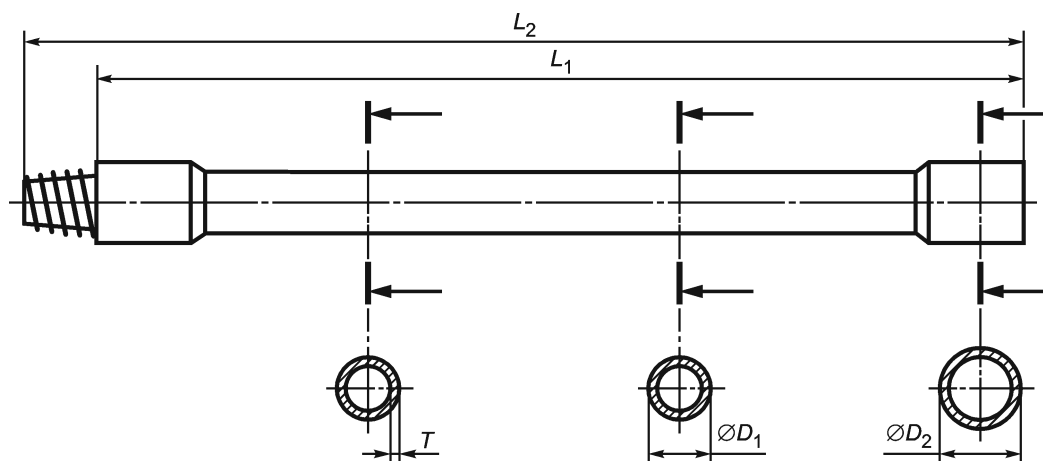
Рисунок 5 — Бурильная труба
