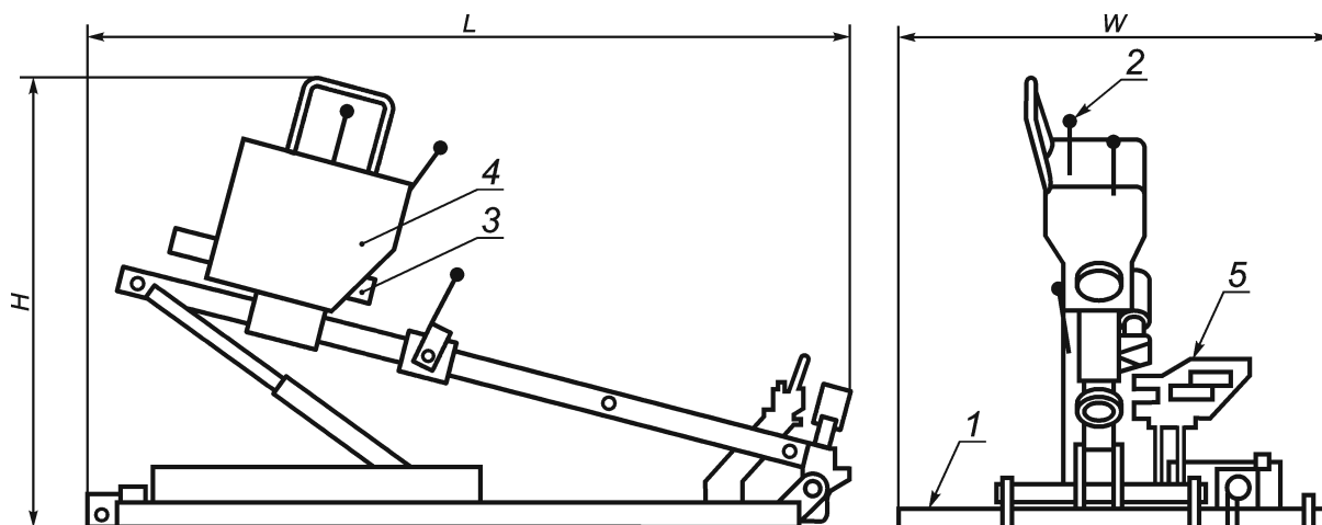
H — общая высота машины; L — общая длина машины; W — общая ширина машины; 1 — место оператора; 2 — управление процессом бурения; 3 — шпindelь; 4 — каретка; 5 — зажим
